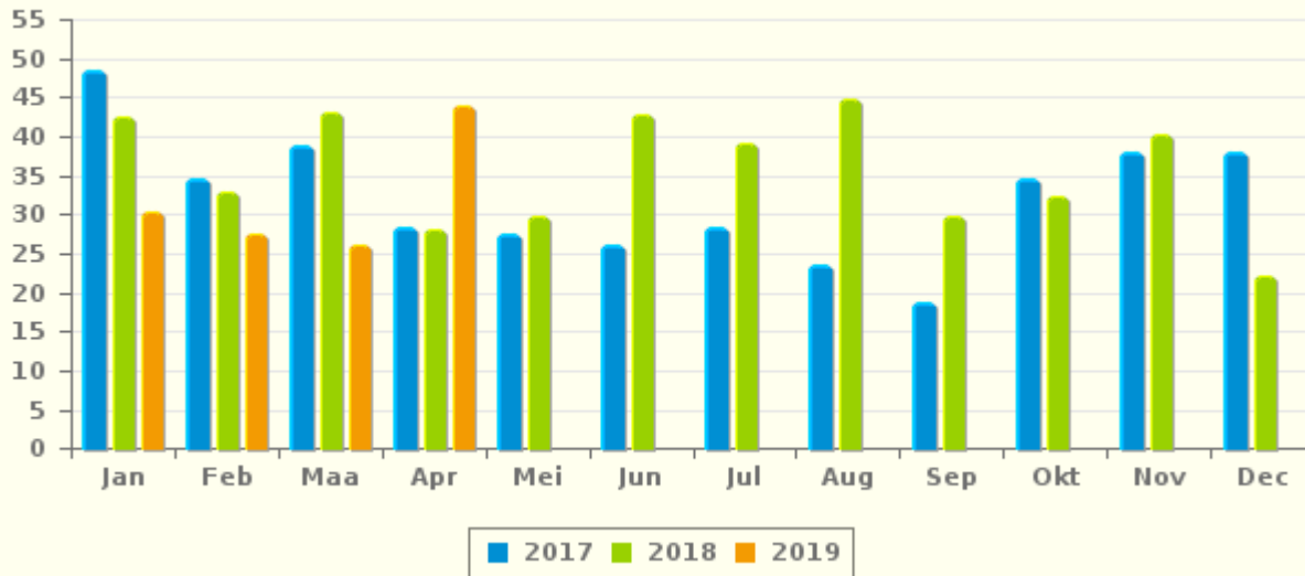
Evolutie van % voertuigen boven getolereerde snelheid (Bemande cont...
